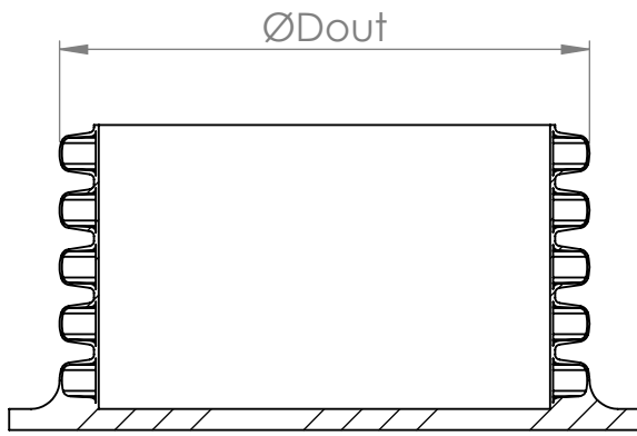
SECTION D-D
