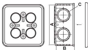
CONDUR® IAR με ίσιες τάπες
